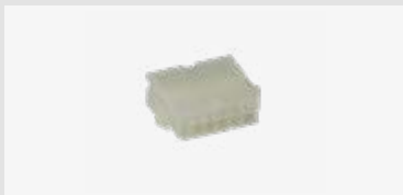
Gehäuse Molex Mini Fit Buchse 12Pin(m) 1 Stück lose
